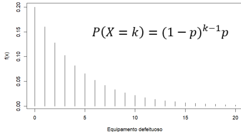
Geométrica (p sucesso = 0.2)
