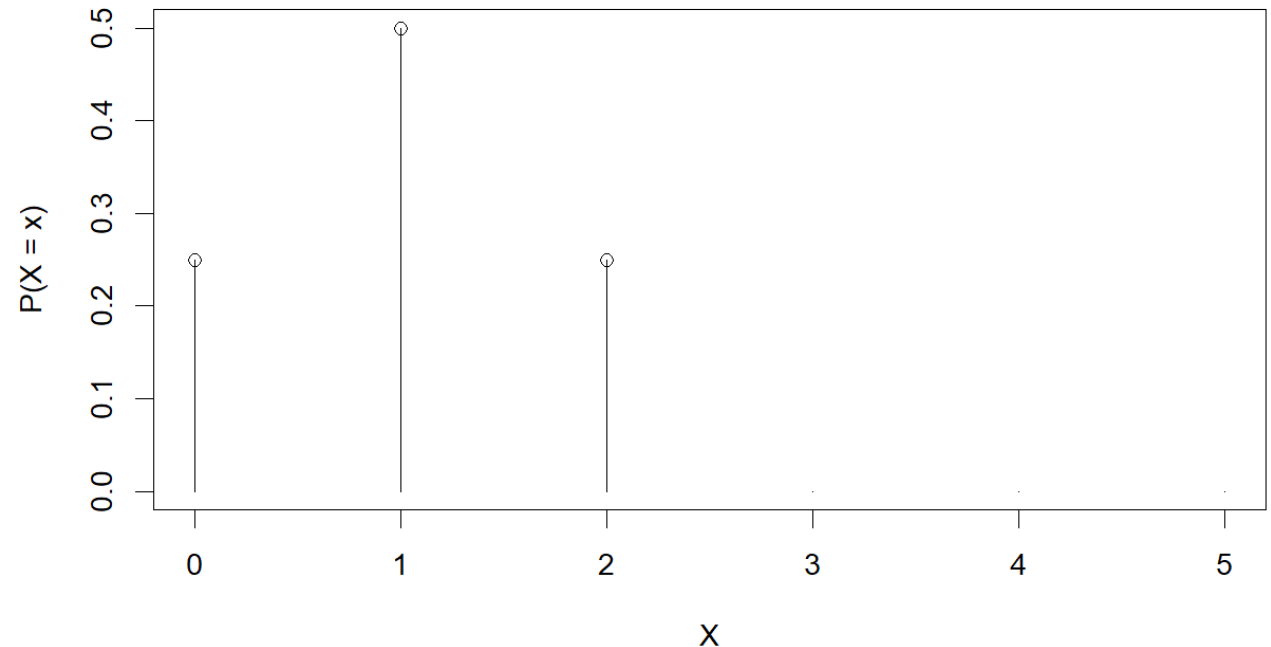
Distribuição de probabilidade da v.a. X
