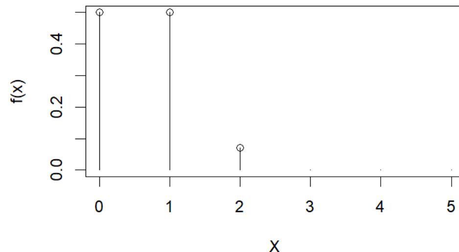
Função de probabilidade
